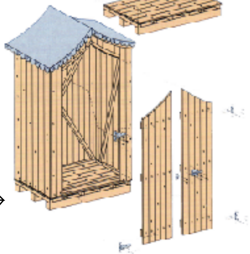
Eclaté de cabane
